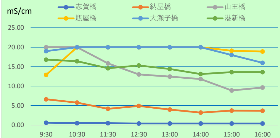
2021 下げ潮 EC(電気伝導度)
