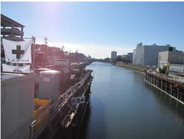
瓶屋橋下流両岸の護岸工事
